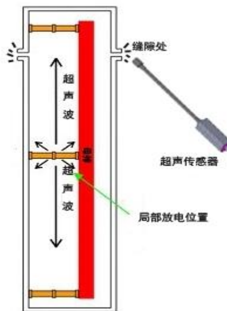
图 3-2 US 测量原理图
