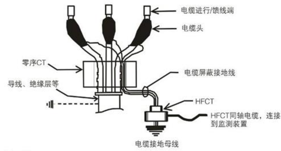
图 3-4 HFCT 测量原理图 2
