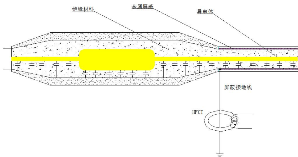
图 3-3 HFCT 测量原理图 1
