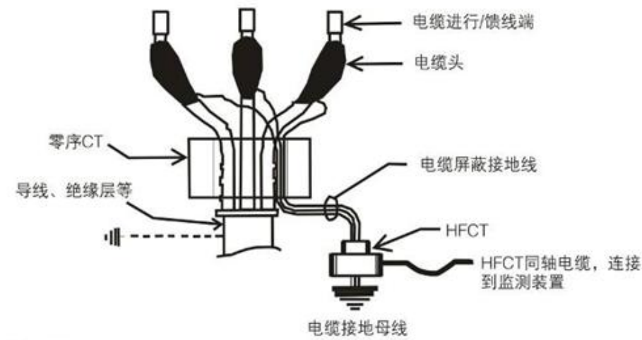
图 3-3 HFCT 测量原理图 2
