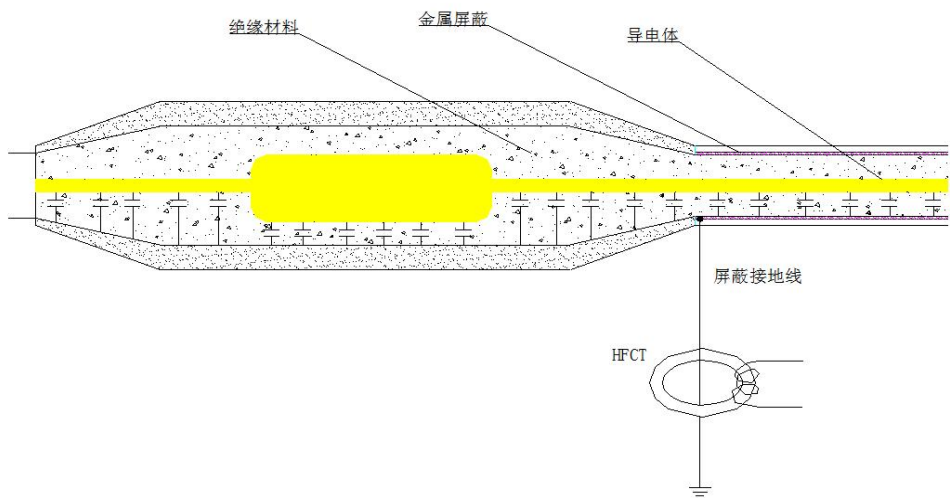
图 3-2 HFCT 测量原理图 1
