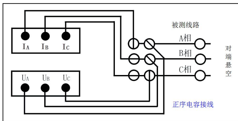
图 5—6、正序电容接线
