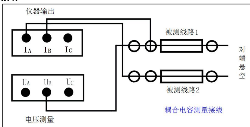
图 5—8、耦合电容接线
