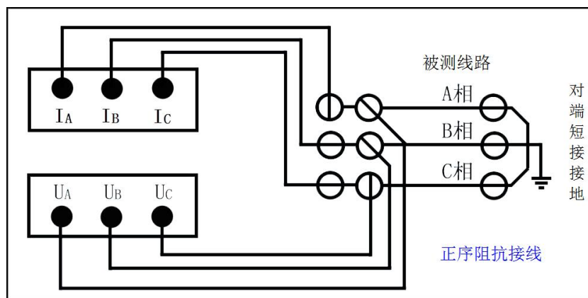
图 5—3、正序阻抗接线
