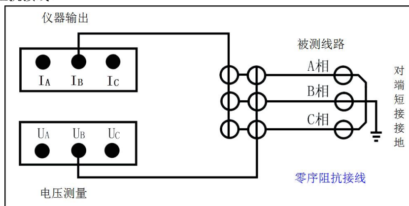
图 5—4、零序阻抗接线
