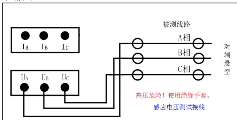
图 5—1、感应电压测试接线
