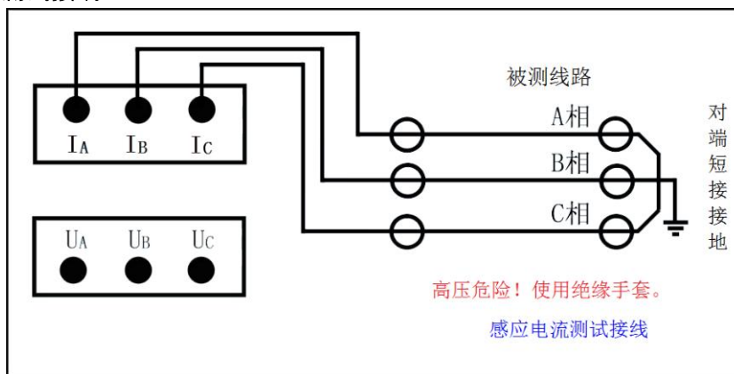
图 5—2、感应电流测试接线
