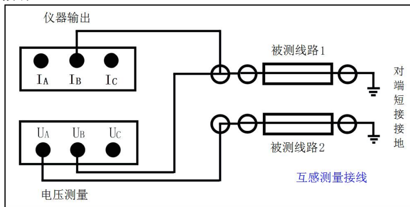
图 5—5、线路互感接线
