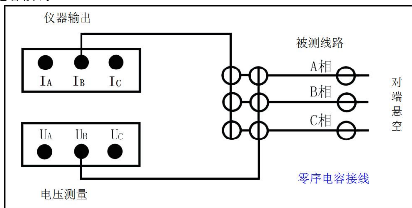
图 5—7、零序电容接线
