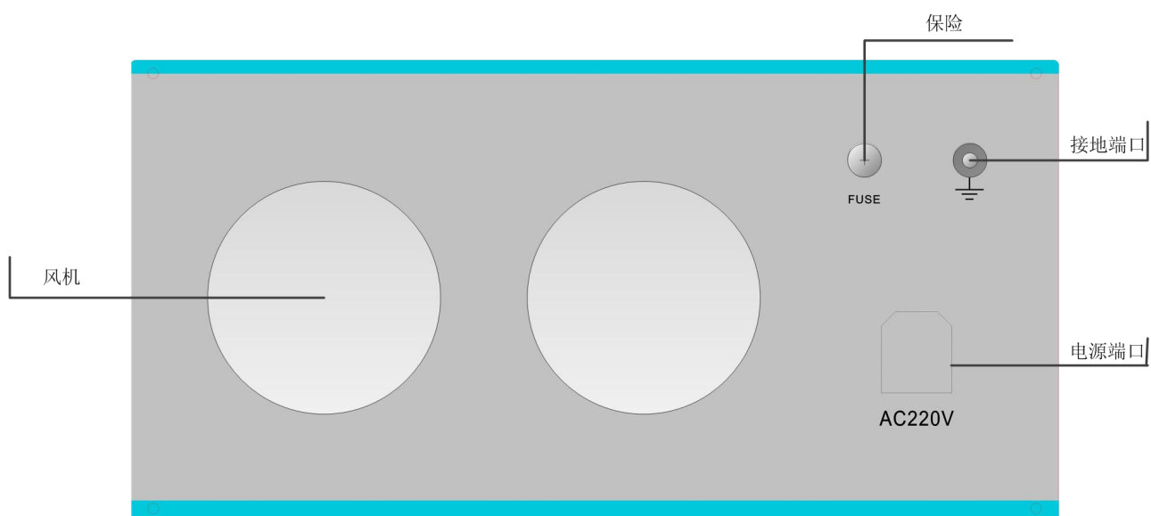
后面板布局示意图
