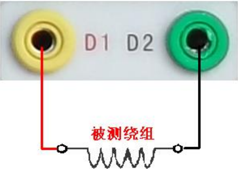
图 37，直阻测试接线图
