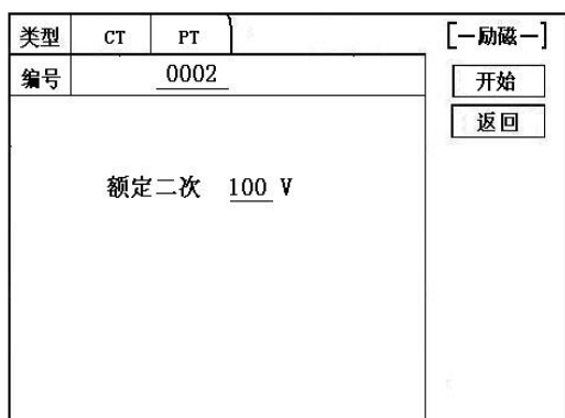
图 24，PT 励磁特性参数设置界面
