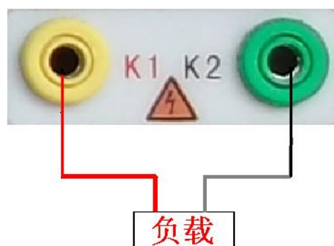
图 20，CT 二次负荷接线图
