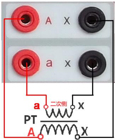
图 28 ，PT 变比极性（角差比差）接线图
