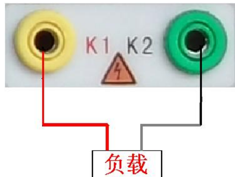
图 34，CT 二次负荷接线图
