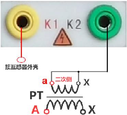
图 32，PT 交流耐压接线图
