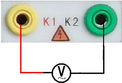
图 42，电压校准接线图
