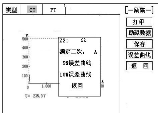
6，CT 励磁曲线图
