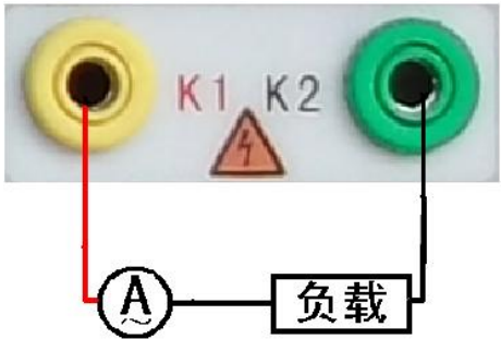
图 43，电流校准接线图
