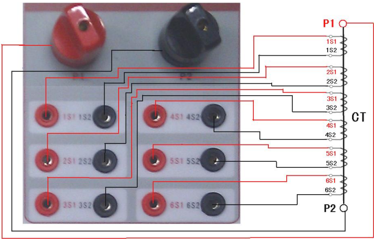
图 10 ， CT 变比极性（角差比差）接线图
