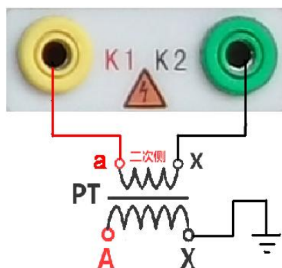
图 25，PT 励磁特性接线图
