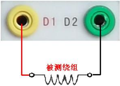
图 23，直阻测试接线图
