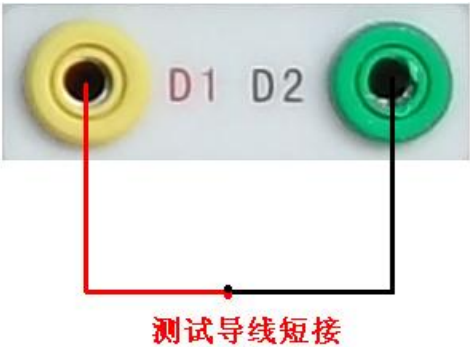
图 36，导线阻值清零接线图
