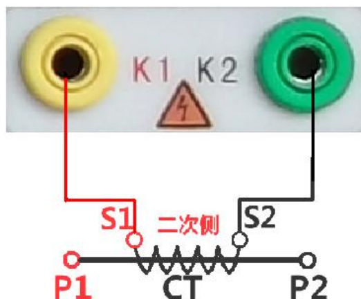
图 5，CT 励磁特性接线图
