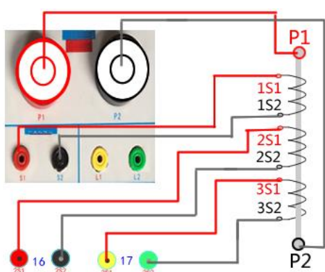
图 14， 电流法 CT 变比极性 （角差比差）接线图
