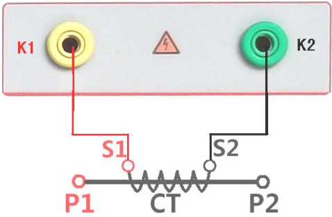
图 5，CT 励磁特性接线图
