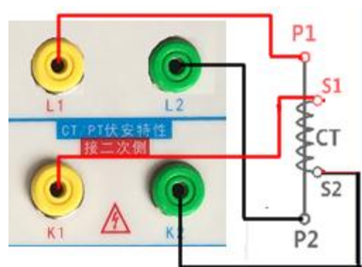
图 15， 电压法 CT 变比极性 （角差比差）接线图
