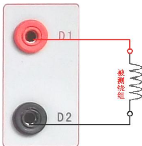
图 26，直阻测试接线图
