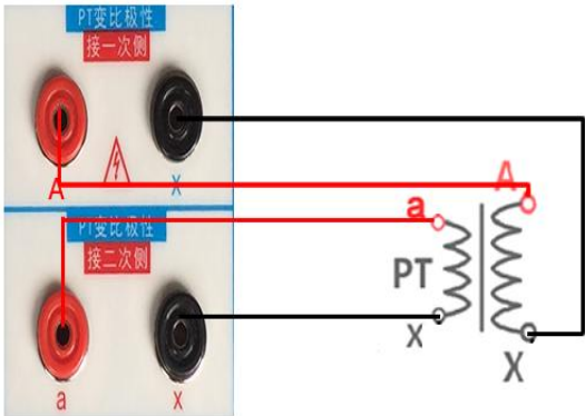
图 31，PT 变比极性（角差比差）接线图
