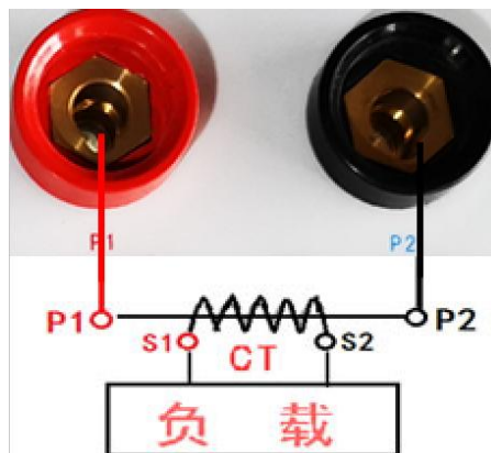
图 19、CT 一次通流接线图
