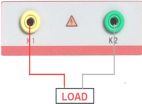
图 37，PT 二次负荷接线图
