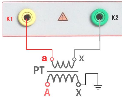
图 28, PT 励磁特性接线图
