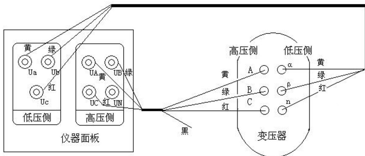
图二十四、斯科特型变的测试接线
