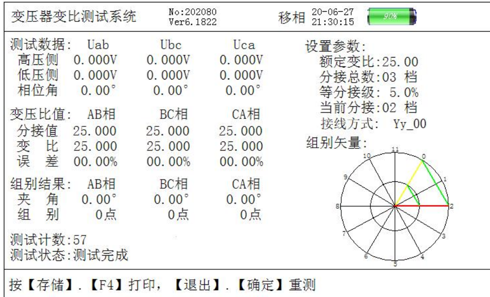
图二十、低压变测试结果屏
