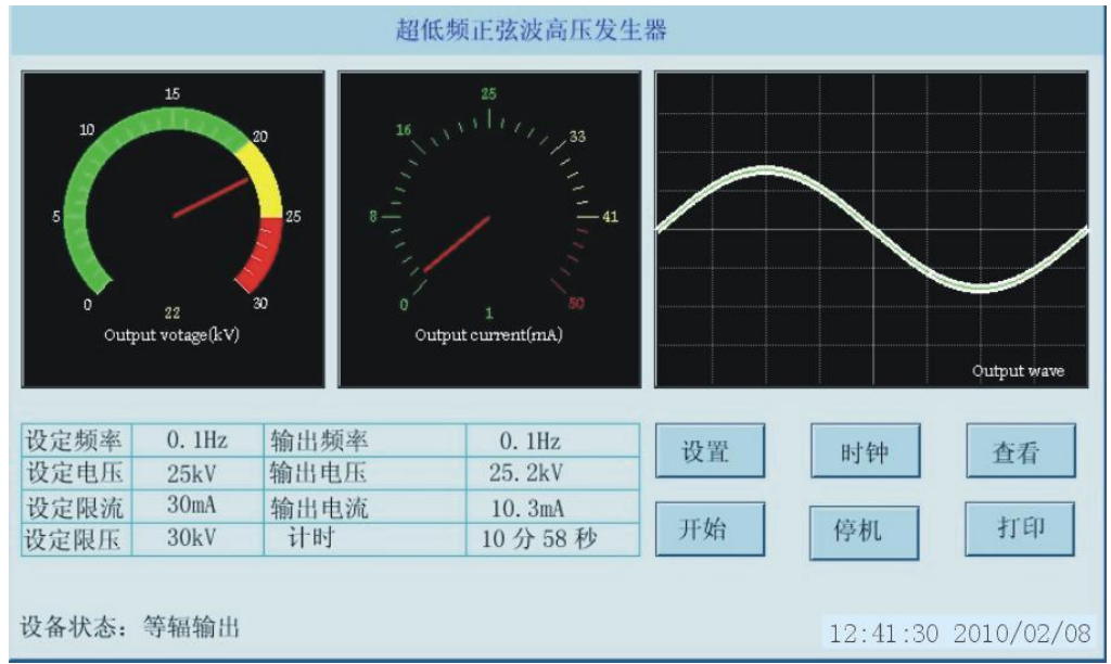
图 8 控制器提示等幅输出
