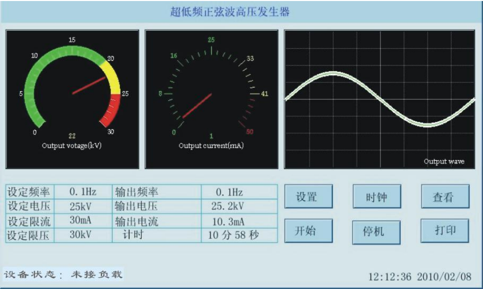
图 6 控制器提示未接负载
