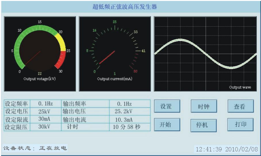
图 10 控制器提示正在放电
