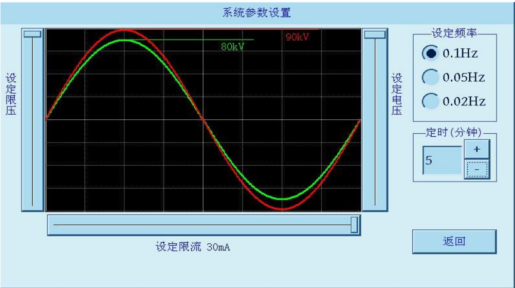
图 5 参数设置界面
