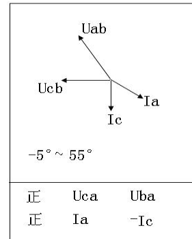
A、B、C三相电压顺序接错
